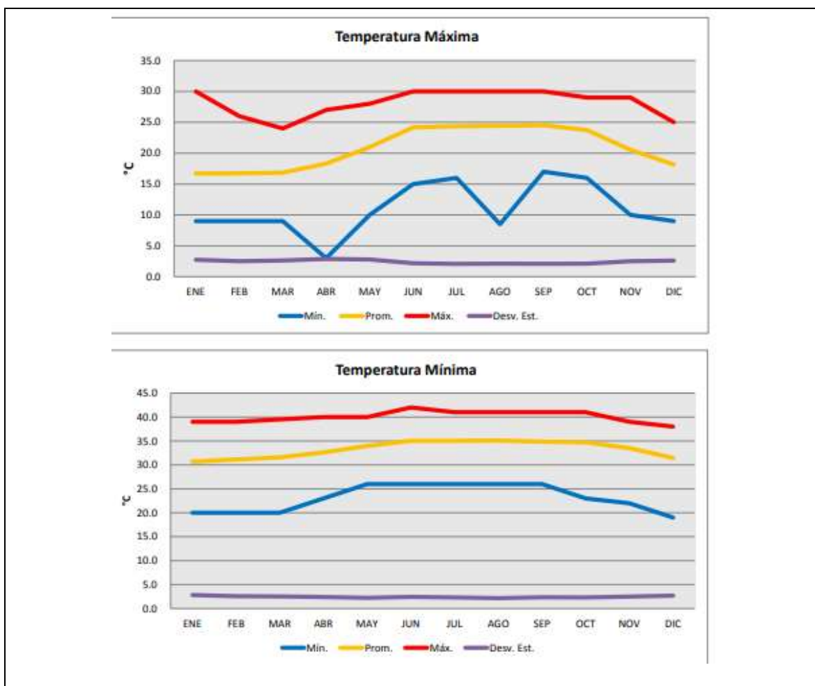
Ilustración 4-Temperatura mensual promedio de la estación climatológica San José
