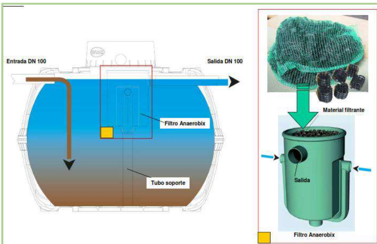
Ilustración II.2 Funcionamiento del biodigestor
