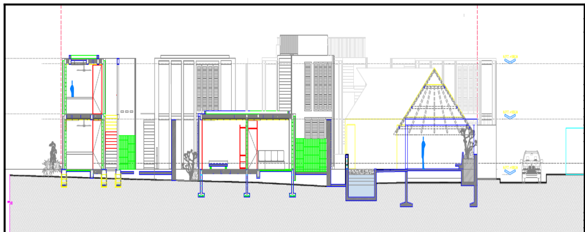
Imagen 13. Corte transversal del proyecto.
