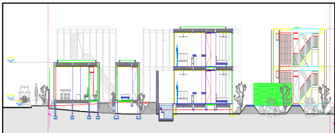
Imagen 14. Corte longitudinal del proyecto.
