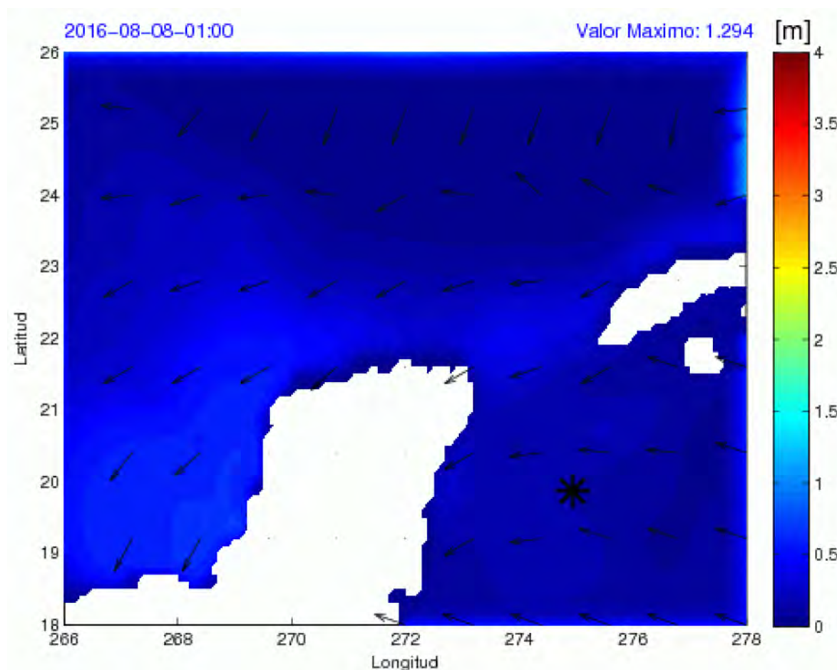
Figura IV:16. Modelación de viento y oleaje del Mar Caribe y Golfo de México. Fuente: Instituto Mexicano de Tecnología del Agua, 28 de agosto de 2016; en línea: http://ciclón.imta.mx/oleaje/
