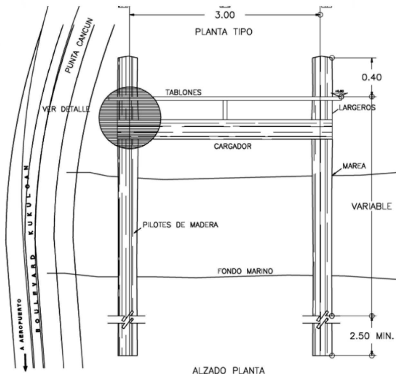
Figura II:12. Detalle constructivo de los pilotes de madera de la Marina Flamingo.
