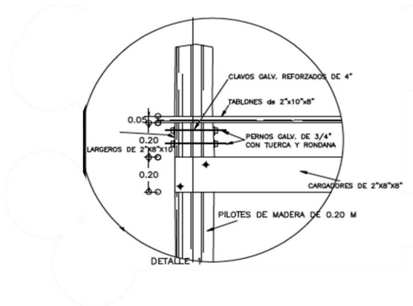
Figura II:10. Detalle constructivo de los pilotes de la Marina Flamingo
