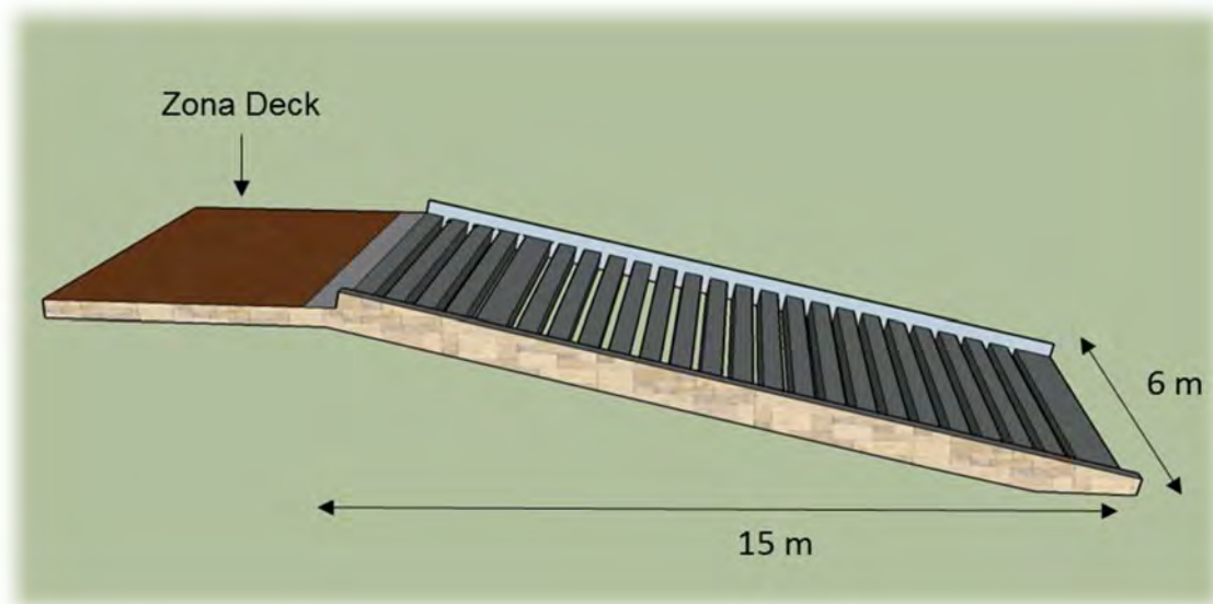
Figura II:11. Vista Perfil de rampa de concreto del Proyecto Marina Flamingo
