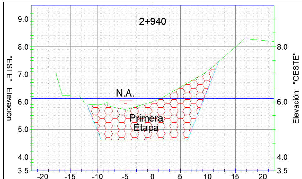
Imagen 7.-Sección de extracción típica.
