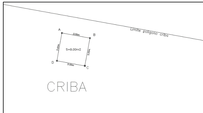
Imagen 14.-Dimensiones del Almacén de Temporal de Residuos Peligrosos.
