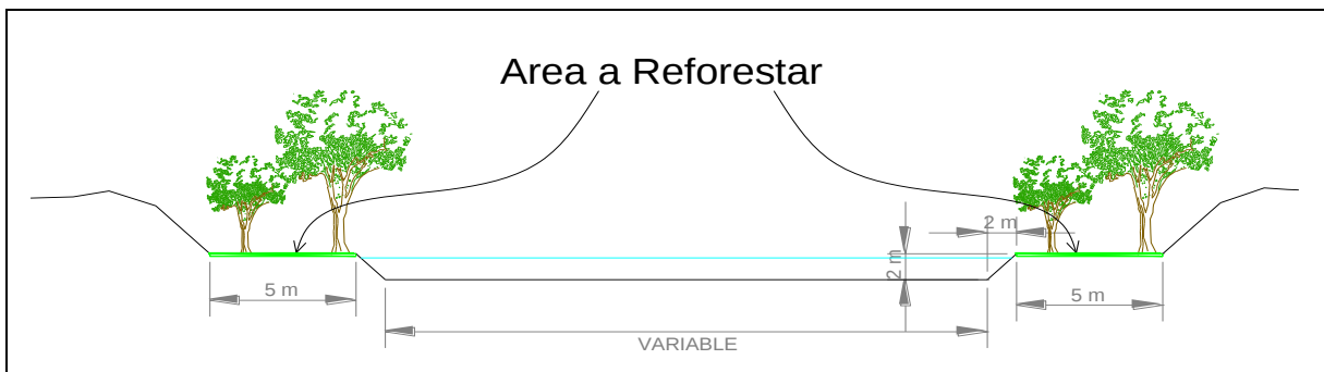
Imagen 10.-Sección tipo del cauce con el proyecto finalizado.
