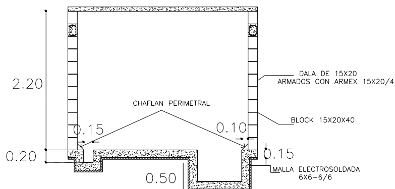
Imagen 13.-Diseño del almacén temporal de residuos peligrosos.
