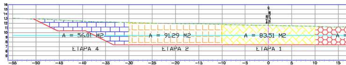
FIGURA 4. ESTACION 0+620.000 (Parte final del proyecto):
