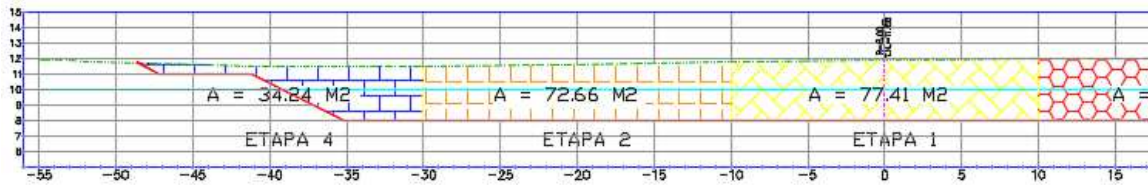
FIGURA 3. ESTACION 0+320.000 (Parte central del proyecto):
