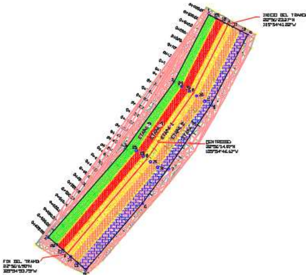
FIGURA 7. 1 SECCION, 5 FRENTES DE EXTRACCIÓN DIVIDIDOS EN 32 ESTACIONES. (PLANO PLANTA DE EXTRACCIÓN)
