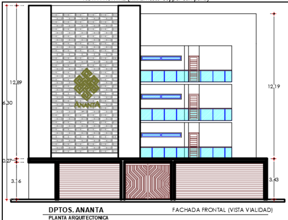
VISTA FRONTAL (Av. Ernesto Coppel Campaña)
