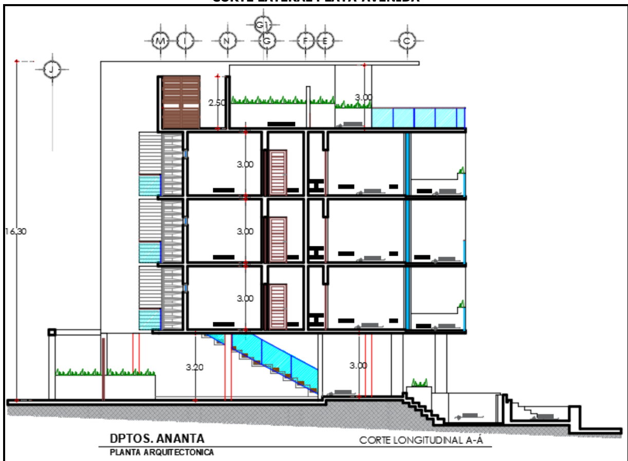
CORTE LATERAL PLAYA-AVENIDA
