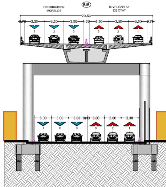
Figura 18. Detalle Km 7+684.00, sección tipo.
