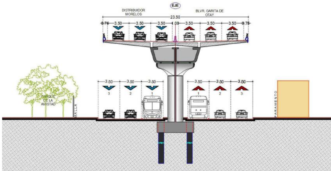
Figura 5. Sección tipo de 6 carriles.
