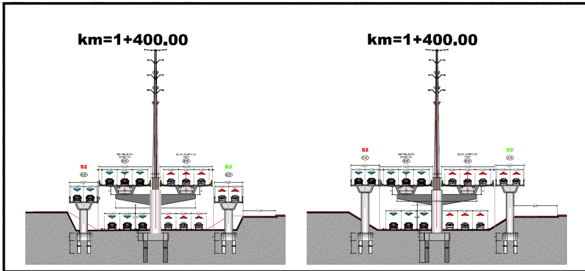
Figura 7. Detalle E2 y S2, sección tipo.
