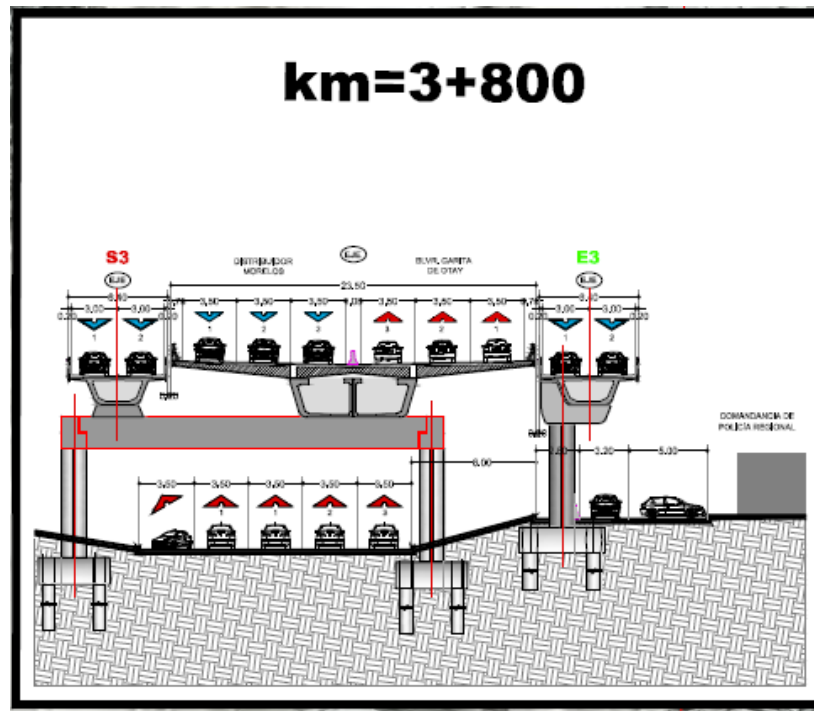
Figura 10. Detalle S4, sección tipo.
