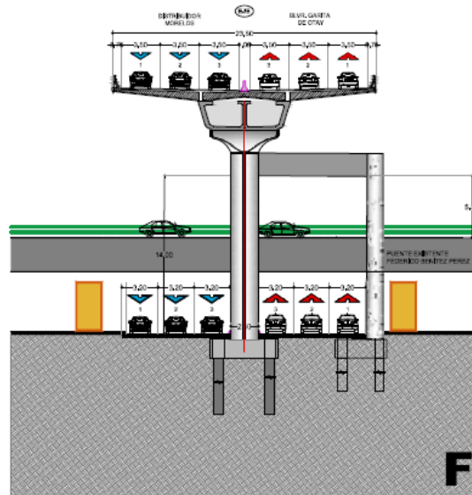
Figura 16. Detalle E5 y E6, sección tipo.
