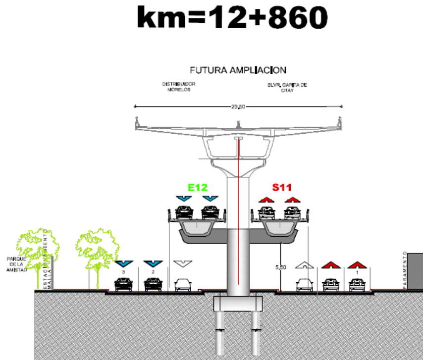
Figura 26. Detalle Km 12+860.00, E12 y S11, sección tipo.
