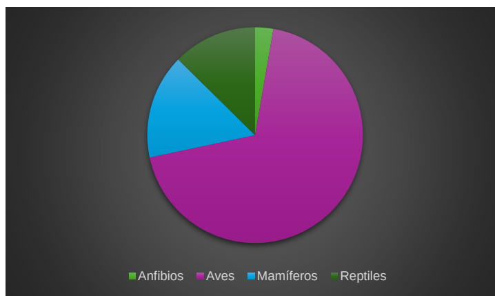
Figura 26. Porcentaje de especies de vertebrados terrestres reportados.
