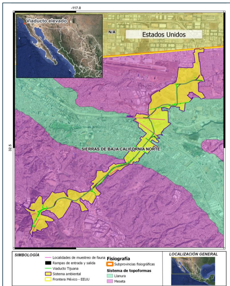
Figura 14. Provincia fisiográfica del SA y AP.
