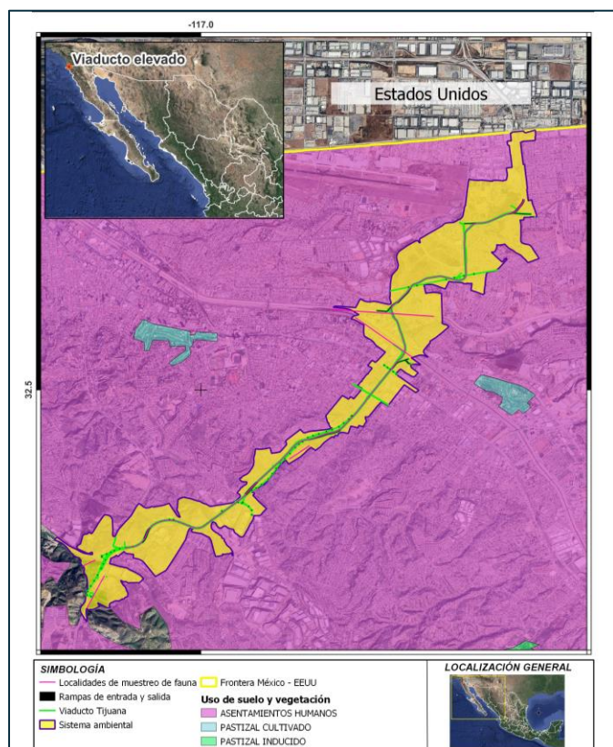
Figura 20. Uso de suelo y vegetación en el SA y AP.
