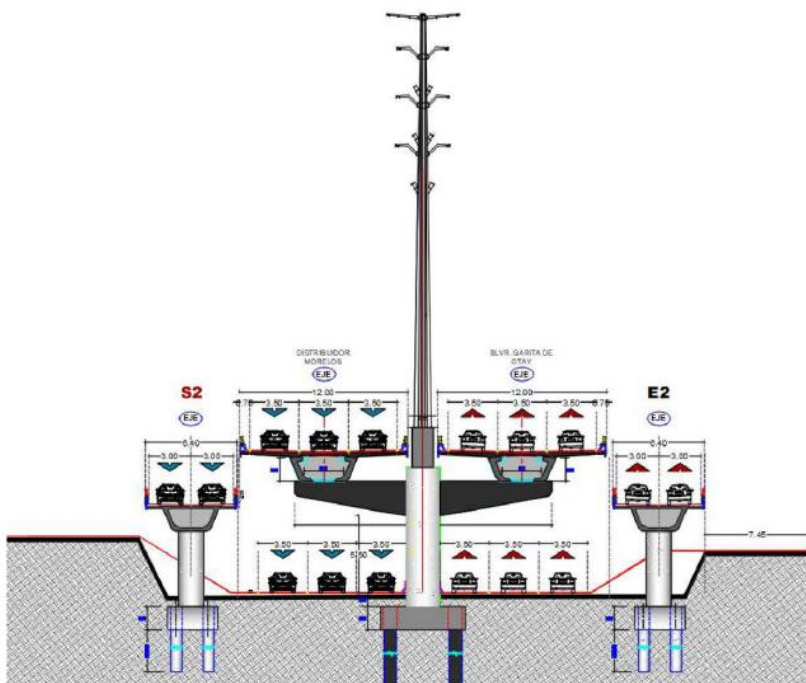
Figura 30. Sección en distribuidor.
