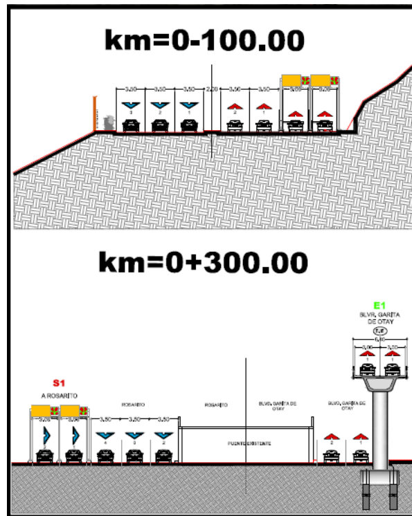
Figura 6. Detalle distribuidor Morelos E1 y S1, sección tipo.
