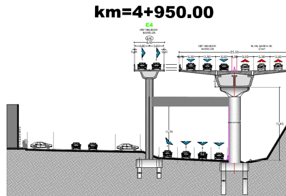
Figura 12. Detalle E5 y E6, sección tipo.
