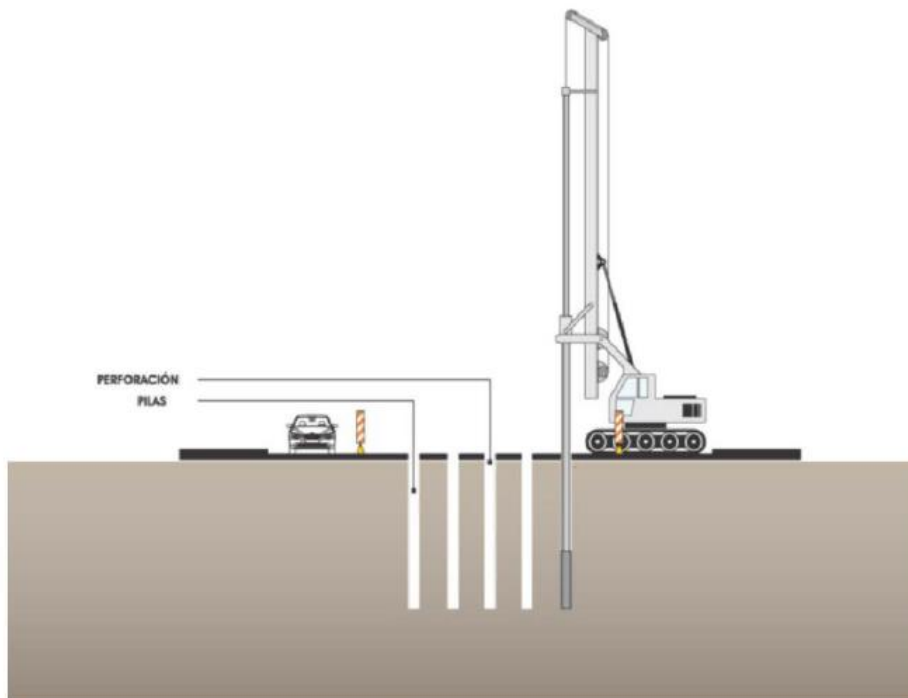
Figura 32. Perforación pilas.
