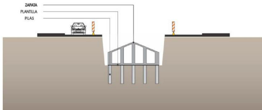
Figura 35. Zapata.
