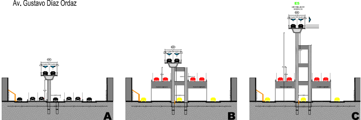
Figura 16. Detalle E5 y E6, sección tipo.
