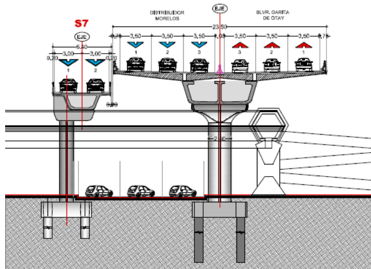
Figura 22. Detalle Km 11+163.00, sección tipo.
