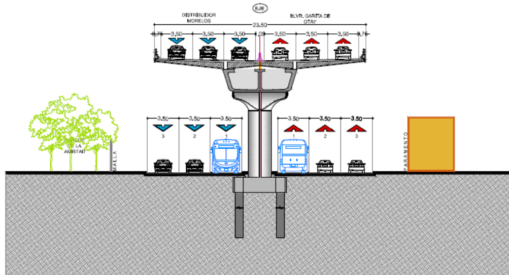
Figura 24. Detalle Km 12+700.00, E12 y S11, sección tipo.
