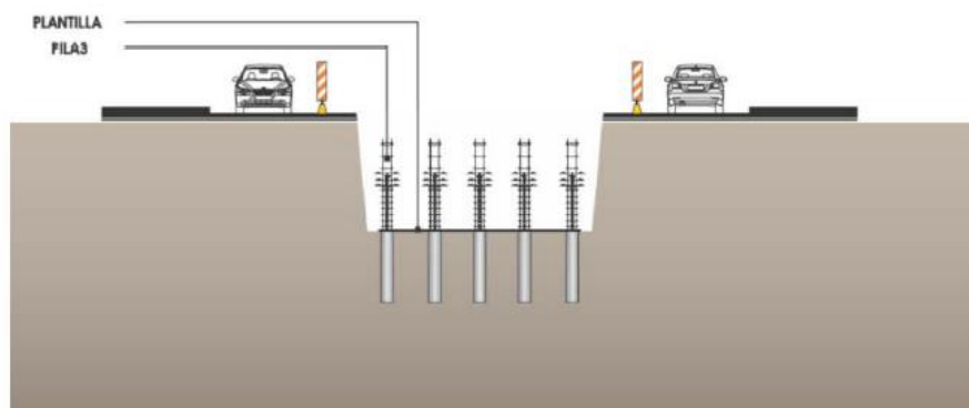
Figura 34. Descabece de pilas.
