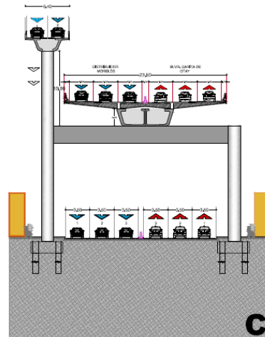
Figura 14. Detalle E5 y E6, sección tipo.
