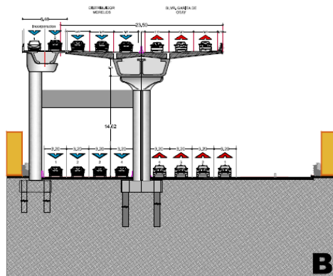
Figura 14. Detalle E5 y E6, sección tipo.
