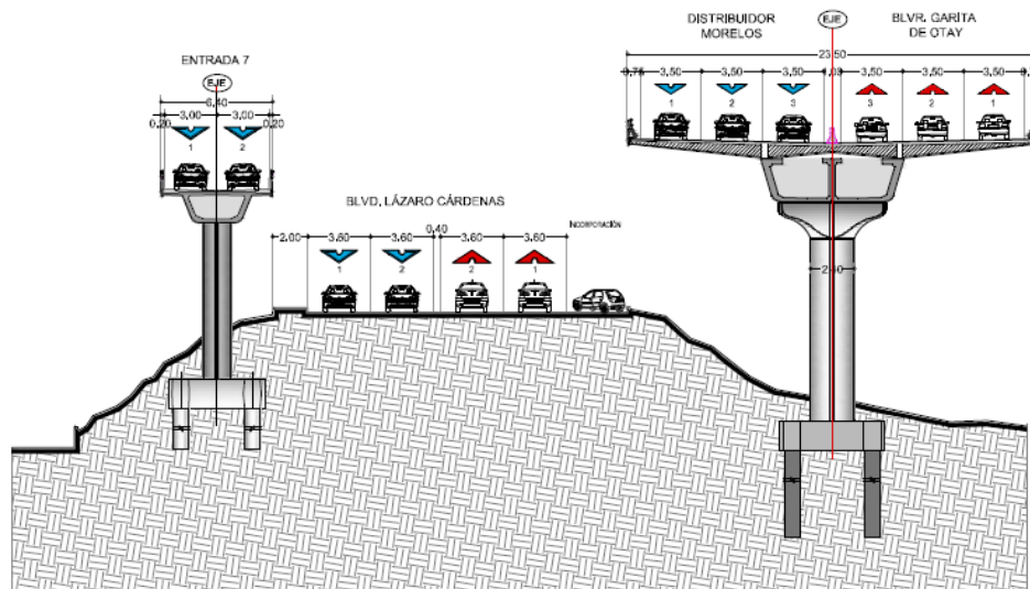
Figura 20. Detalle Km 8+805.50, sección tipo.
