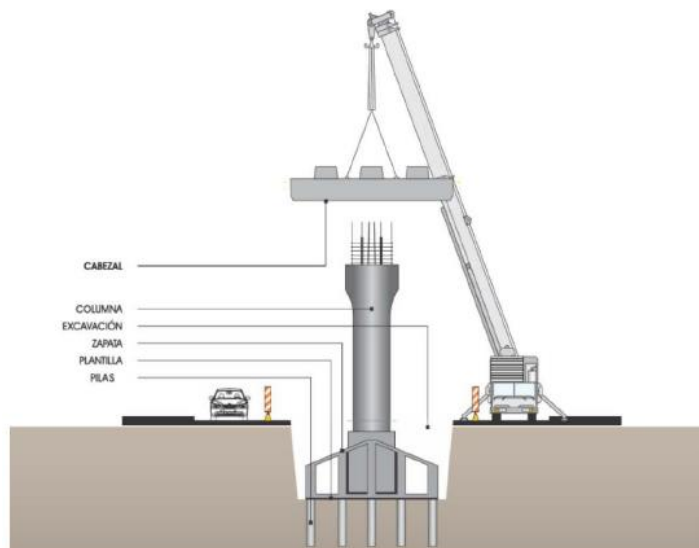
Figura 37. Montaje de cabezal.
