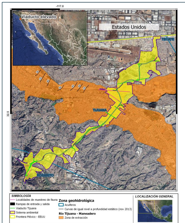
Figura 19. Hidrología subterránea en el SA y AP.
