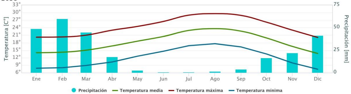
Figura 10. Clima del SA y AP.
