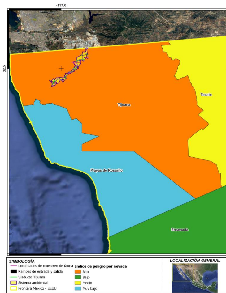
Figura 11. Grado de peligro por nevadas en el SA y AP.
