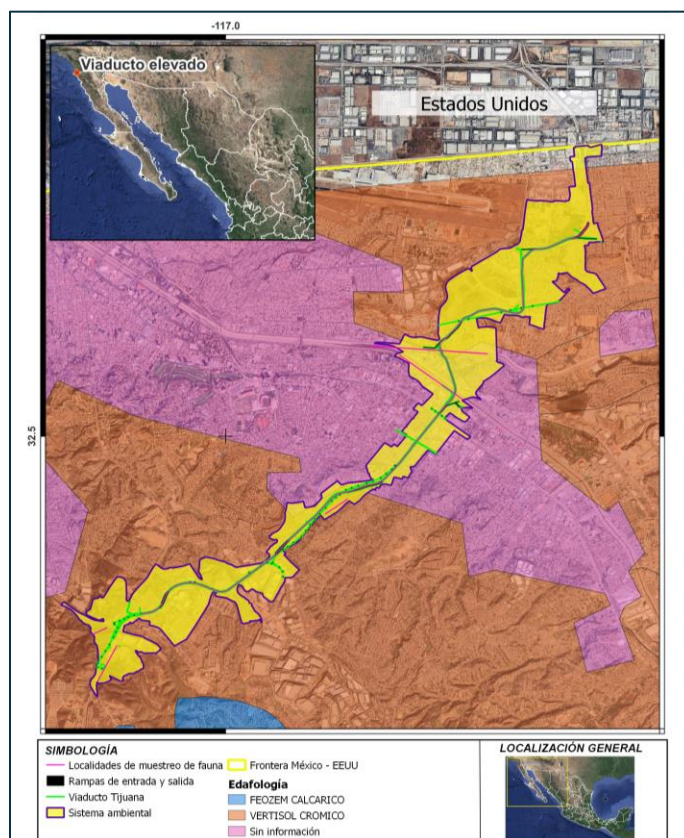
Figura 16. Suelo en el SA y AP.
