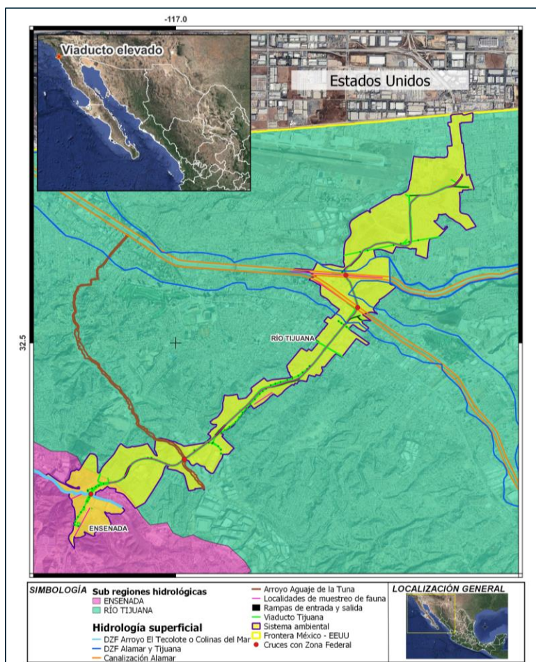
Figura 18. Hidrología superficial en el SA y AP.
