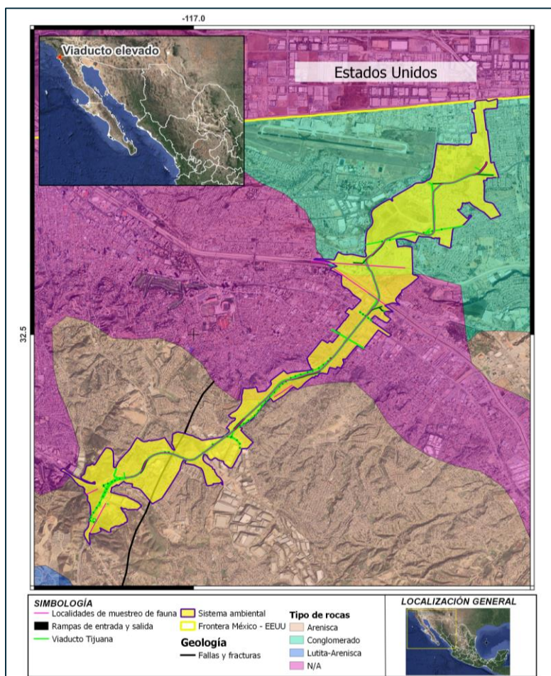
Figura 15. Geología del SA y AP.
