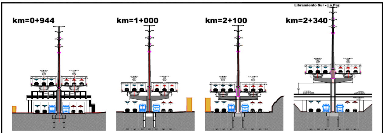
Figura 8. Detalle E2 y S2, sección tipo.
