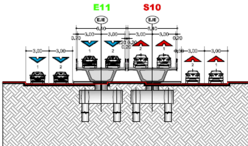
Figura 27. Detalle E11 y S10, sección tipo.
