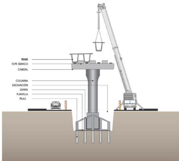
Figura 38. Montaje de trabes.
