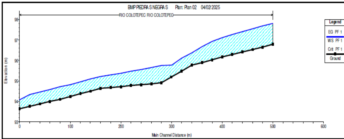
Imagen 4. Perfil del fondo del cauce modificado.
