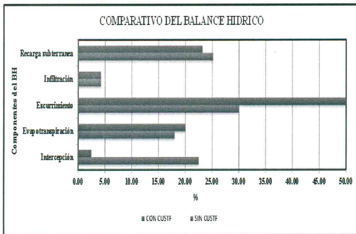
Representación gráfica del balance hidrico nivel proyecto con CUSTF y sin CUSTF.
