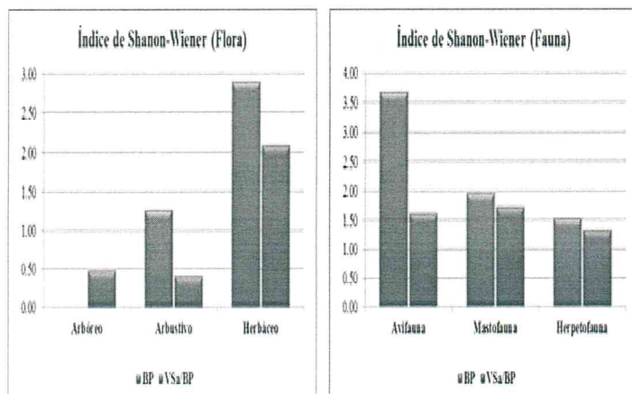
Índice de Shannon-Wiener para los estratos de flora y para los grupos faunísticos en la microcuenca
