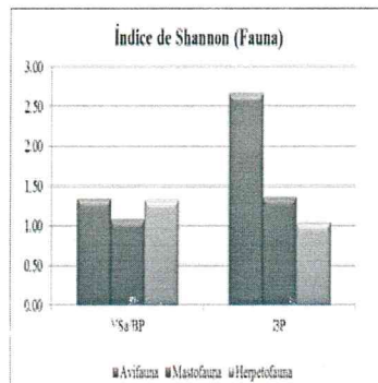
Comparación de índice de Shannon con el software BIODAP (1990)
