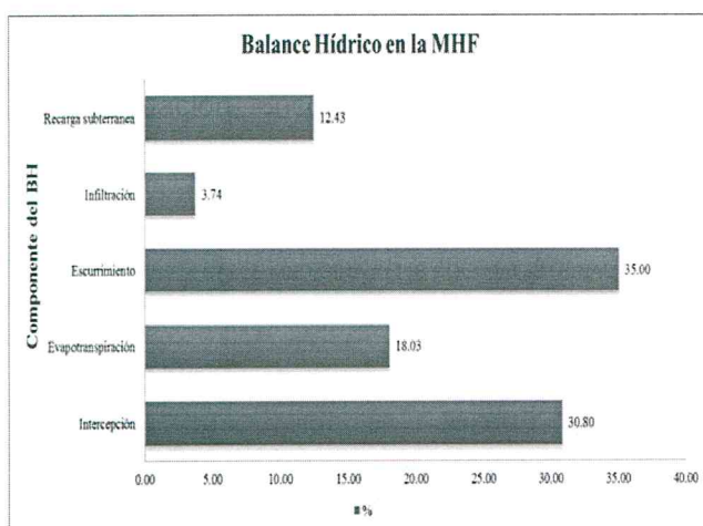
Representación gráfica del balance hídrico nivel microcuenca.
