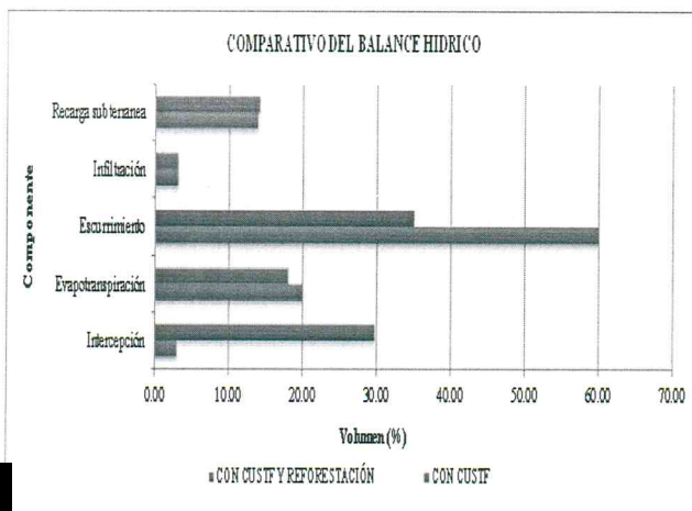
Representación gráfica del balance hídrico con CUSTF y prácticas de reforestación.
