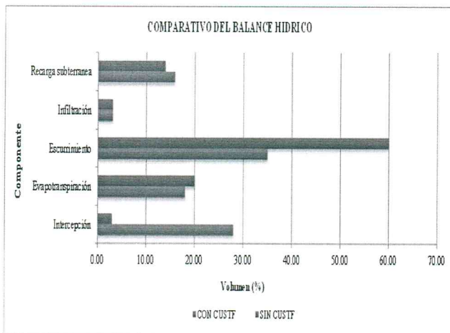
Comparativo del balance hídrico con CUST y sin CUST.
