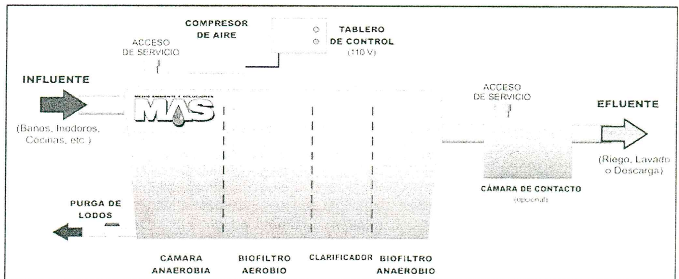
Figura 2. Composición de la planta de tratamiento
