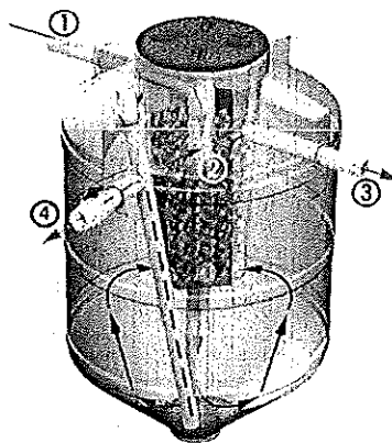
Figura 1.- Funcionamiento del Biodigestor Autolimpiable
