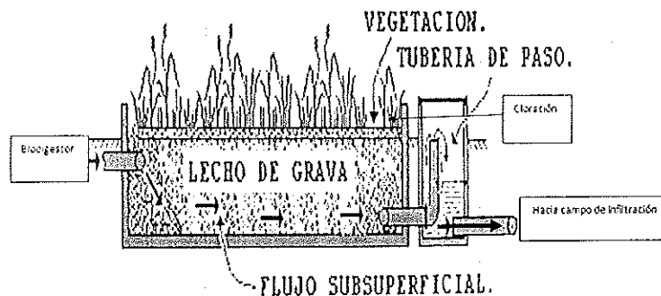
Figura 2. Sistema de tratamiento a base de humedal subsuperficial posterior al biodigestor.
