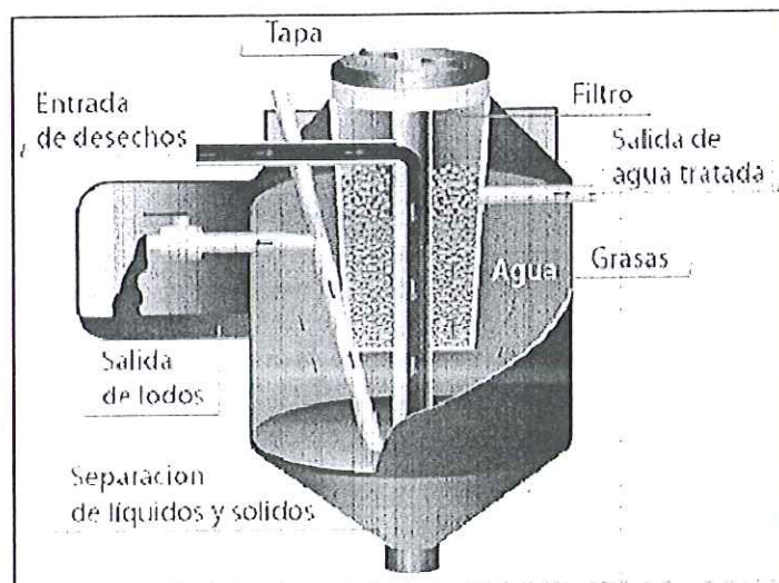
Figura 2.- Componentes del Biodigestor Autolimpiable Rotoplas
