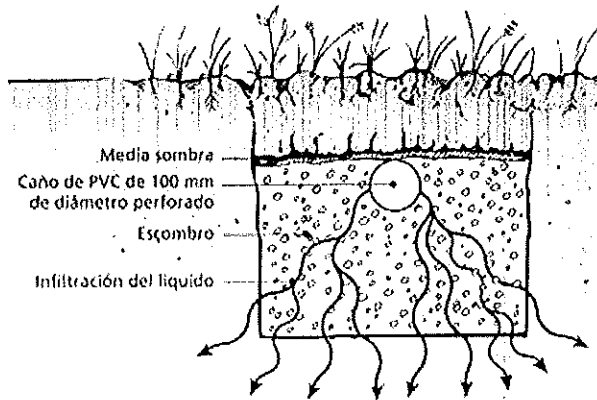
Figura 7. Corte de una sección de la tubería.
