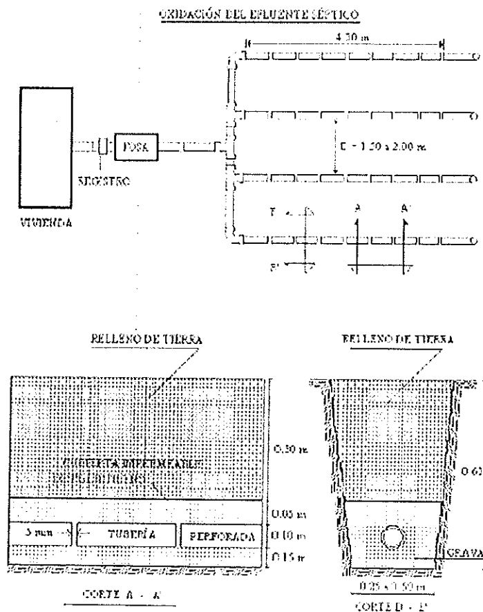
Figura 5. Diagrama general de la dispersión de las zanjas de infiltración.
