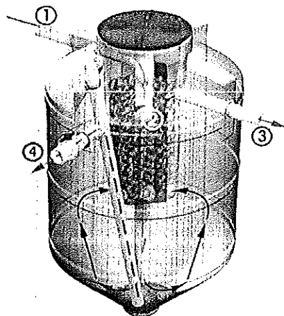
Figura 3.- Funcionamiento del Biodigestor Autolimpiable Rotoplus
