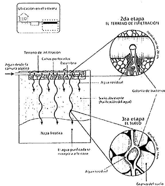
Figura 8. Diagrama del paso de las aguas en las zanjas de infiltración.
