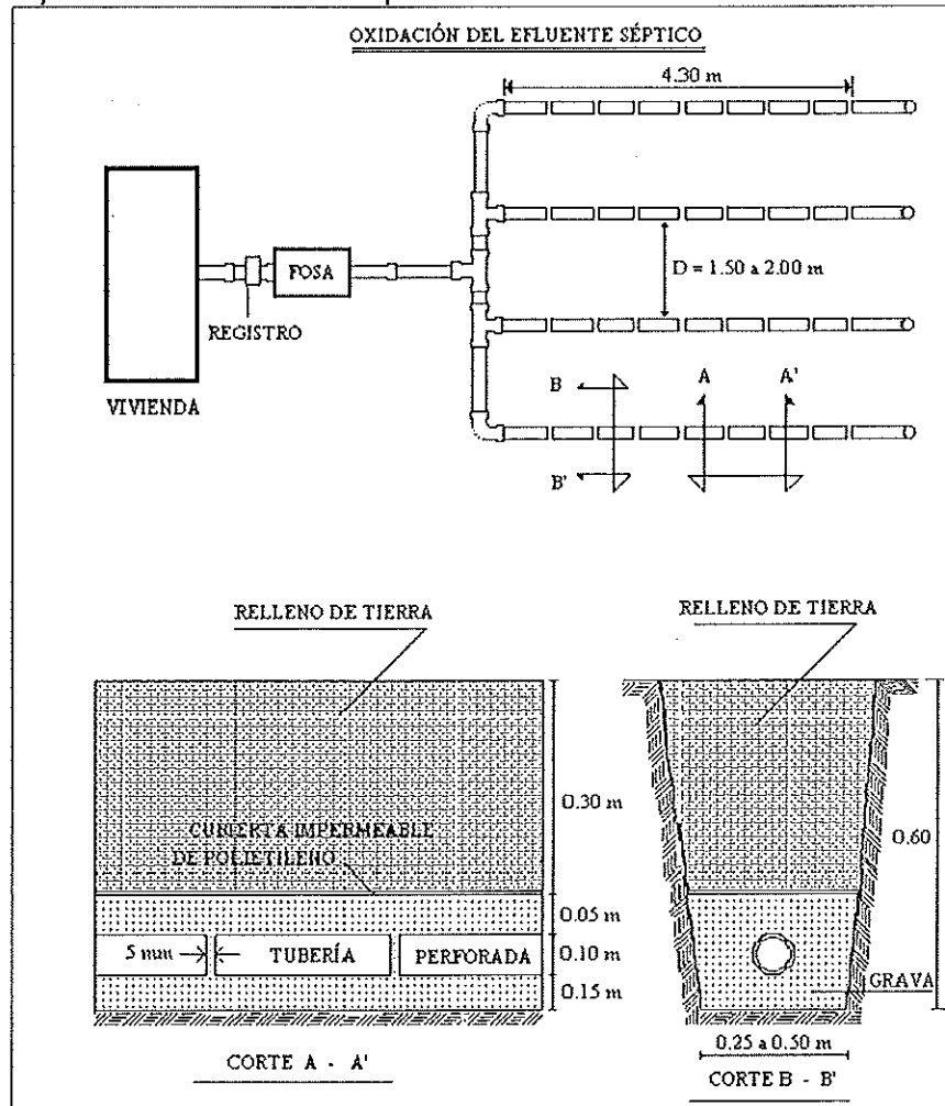
FIGURA 7. ZANJAS DE INFILTRACION (figura ilustrativa)
