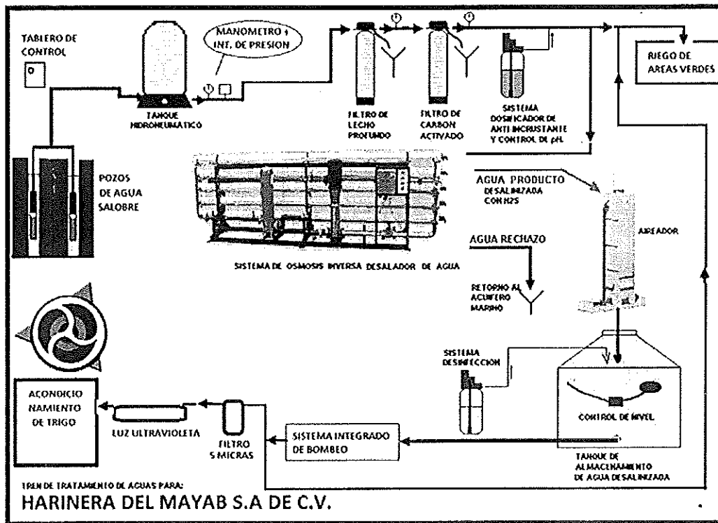
Figura 1.- Diagrama de flujo del sistema de desalinización por ósmosis inversa para el agua utilizada en el proceso de acondicionamiento de trigo.
