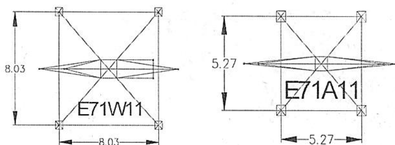
Figura 2.- Área que afectará la cimentación de las estructuras E71W11 y E71A11
