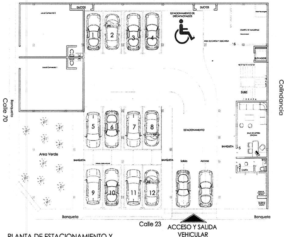
PLANTA DE ESTACIONAMIENTO Y LOCALES Planta Baja
