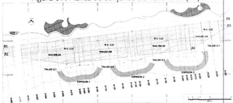
Figura 57. Planta de conjunto del relleno de playa.
