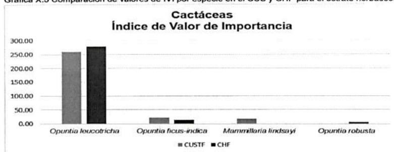
Gráfica X.5 Comparación de valores de IVI por especie en el CUS y CHF para el estrato herbáceo.
