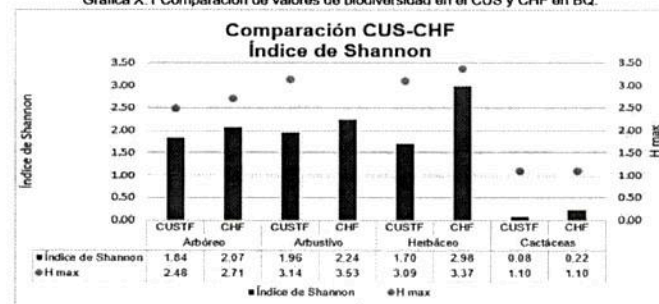
Gráfica X. 1 Comparación de valores de biodiversidad en el CUS y CHF en BQ.
