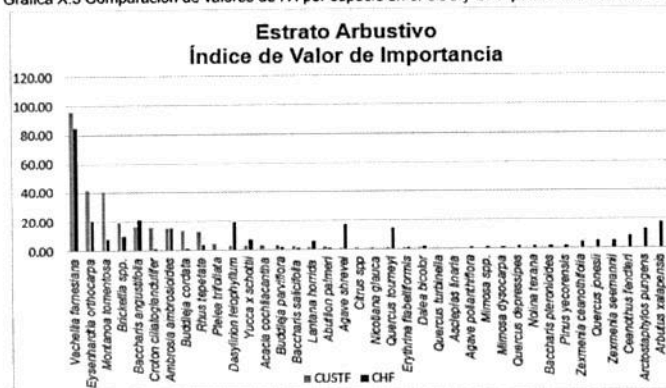
Gráfica X.3 Comparación de valores de IVI por especie en el CUS y CHF para el estrato arbustivo.
