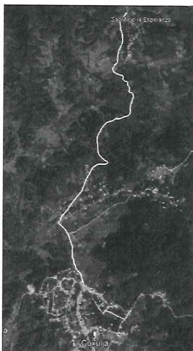
Figura No. 1 Trazo del camino cruce Cuxulja-Ukumilja subtramo del km 0+000 al km 5+000
