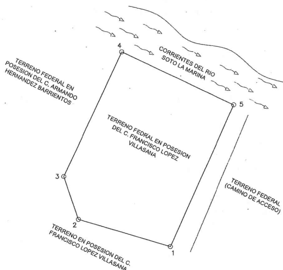
LEVANTAMIENTO TOPOGRAFICO DE UN TERRENO RUSTICO FEDERAL
