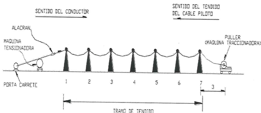
Esquema de las actividades para realizar el tendido del Cable de Guarda con Fibra Óptica CGFO
