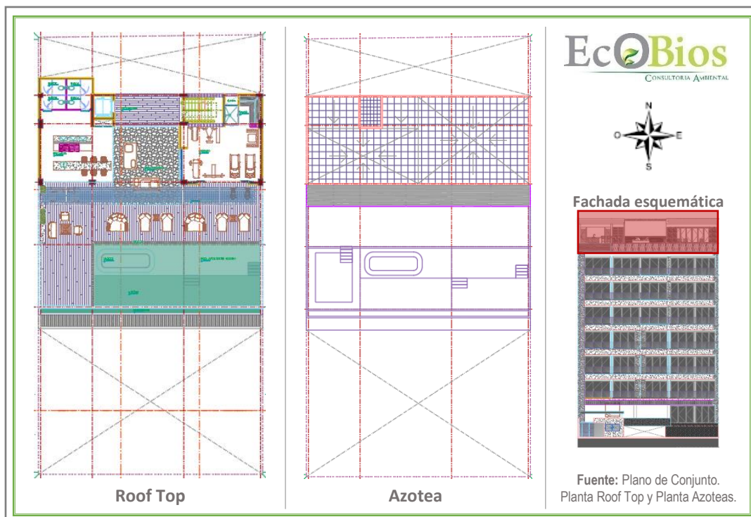
Figura II.5 Detalle del diagrama del polígono del Roof Top y azotea
