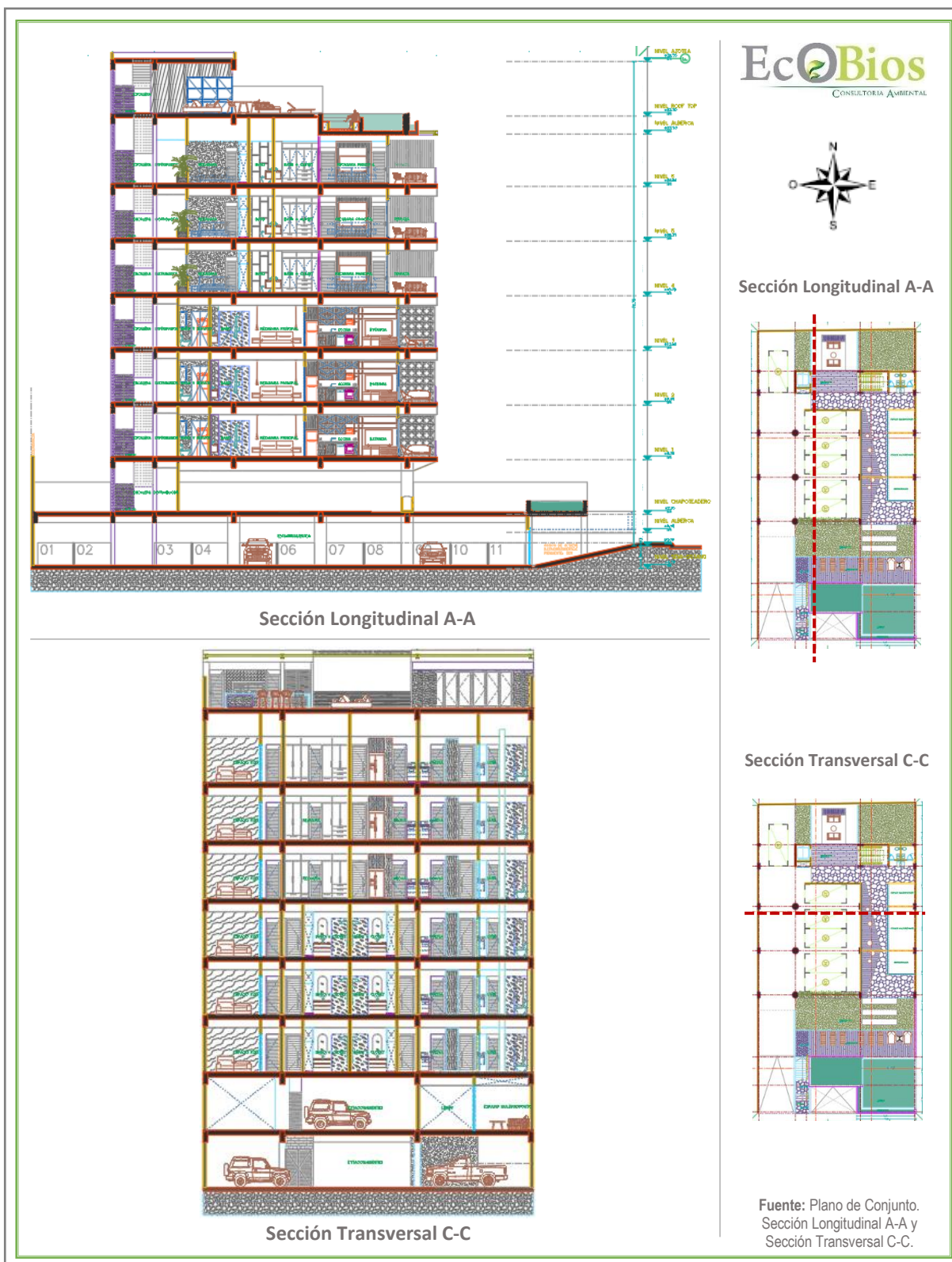
Figura II.6 Muestra el diagrama de las secciones longitudinal y transversal
