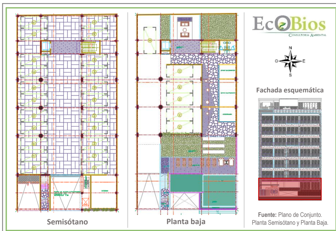
Figura II.3 Detalle del diagrama del polígono del semisótano (área de estacionamiento) y Planta baja (áreas comunes)
