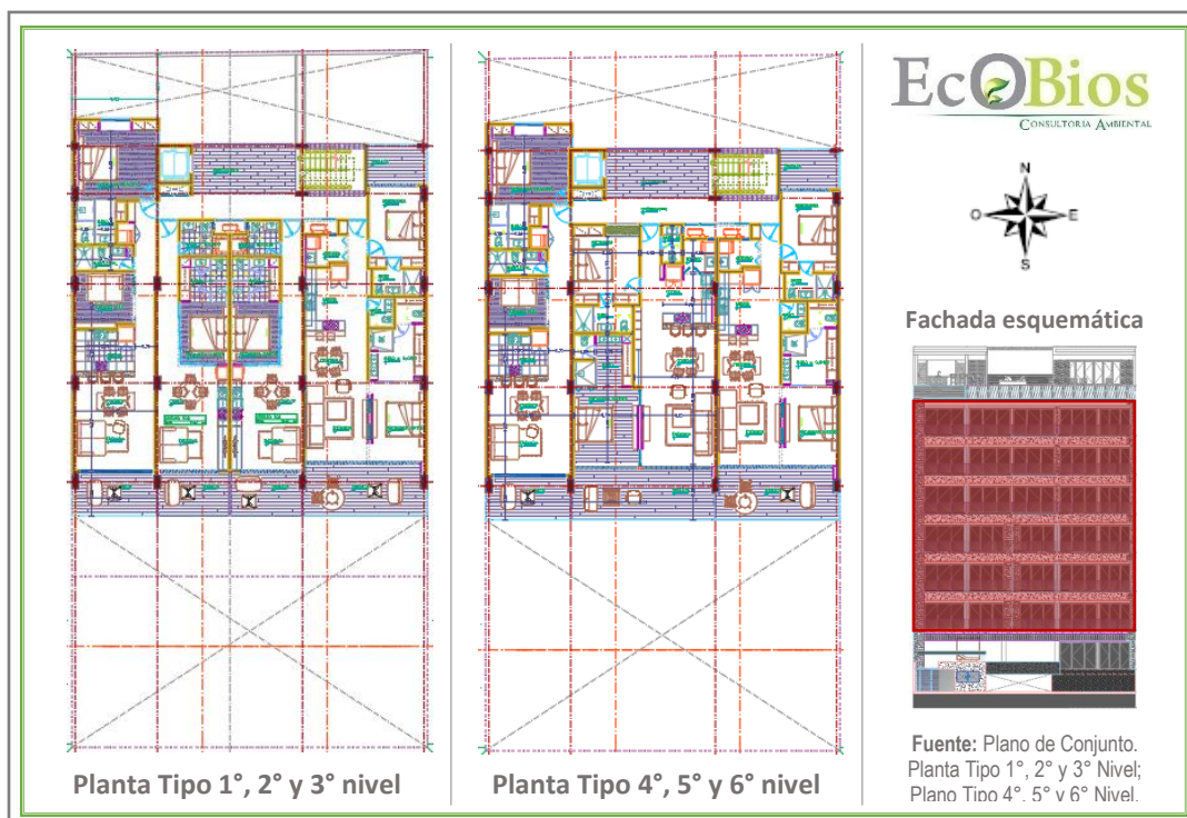
Figura II.4 Detalle del diagrama del polígono del Nivel 1 al 3 y del Nivel 4 al 6 (departamentos)
