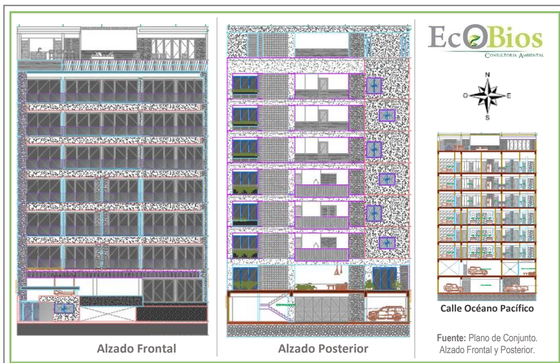
Figura II.7 Vista del alzado frontal y posterior del edificio proyectado
