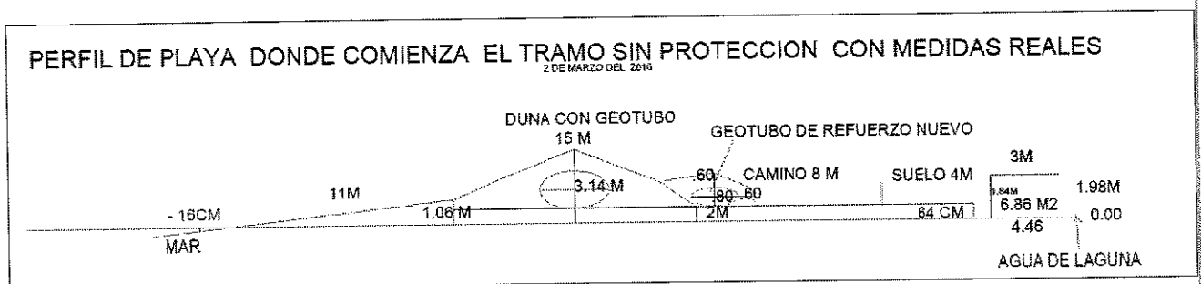
Ilustración 1. Perfil de la playa
