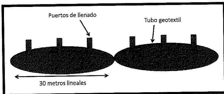
Ilustración 2. Posición de tubos geotextiles durante el llenado.
