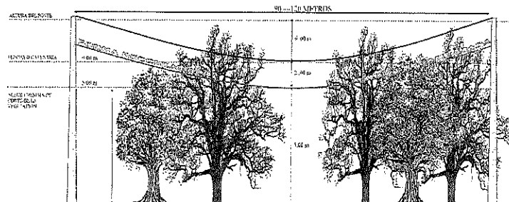
Figura 3.- Las actividades de Poda selectiva deben considerar solo el retiro de las ramas en contacto o próximas al conductor, permitiendo el desarrollo de las ramas que no interfieran con la seguridad de la línea
