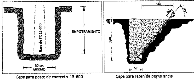
Cepa para poste de concreto 13-600
