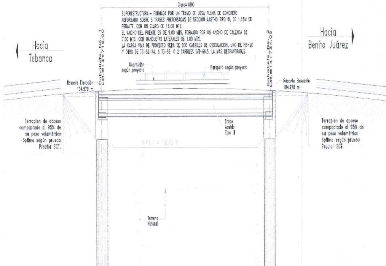
Imagen: Diseño subestructura Estribos y traveses AASHTO III.
