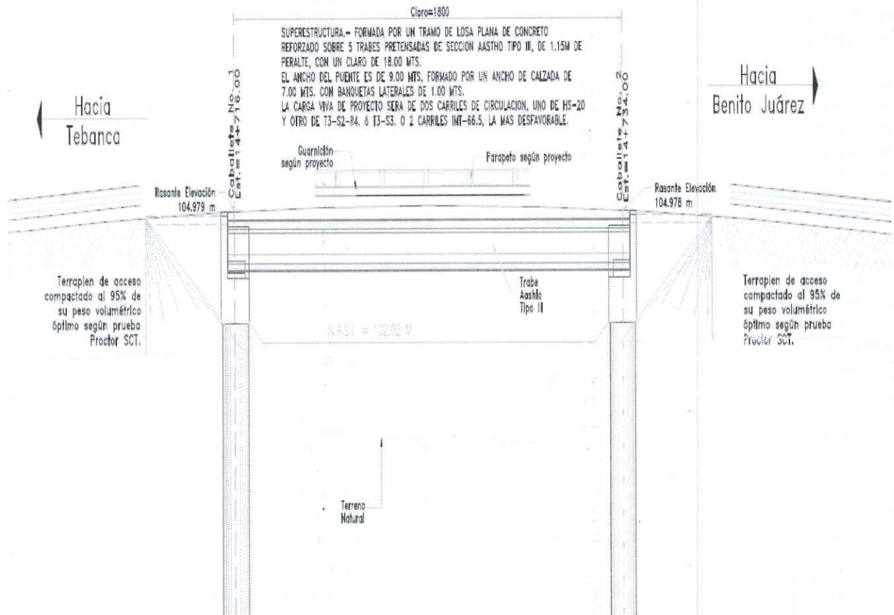
Imagen: Diseño subestructura Estribos y traves AASHTO III.
