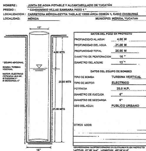
CROQUIS DEL POZO PROFUNDO No. 1
