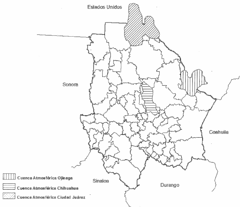
Figura 1. Cuencas atmosféricas del Estado de Chihuahua.
