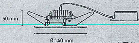
DIMENSIONES
