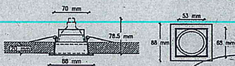
DIMENSIONES
