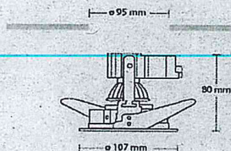
DIMENSIONES
