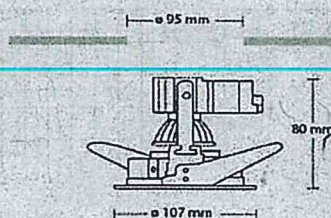
DIMENSIONES
