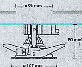
DIMENSIONES
