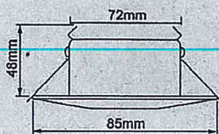
DIMENSIONES
