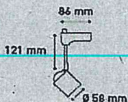
DIMENSIONES
