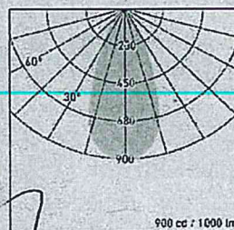
FOTOMETRIAS
