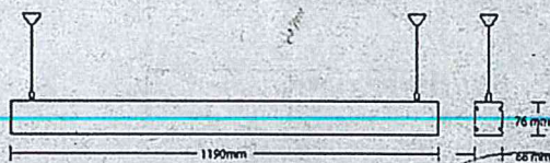
DIMENSIONES
