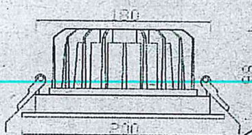
DIMENSIONES
