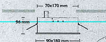
DIMENSIONES
