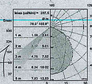
FOTOMETRIAS
