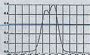
FOTOMETRIAS
