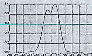
FOTOMETRIAS
