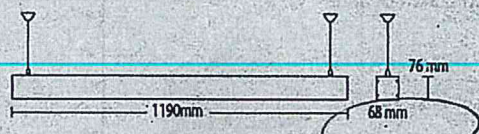
DIMENSIONES
