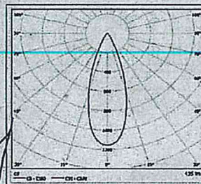
FOTOMETRIAS
