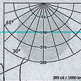
FOTOMETRIAS
