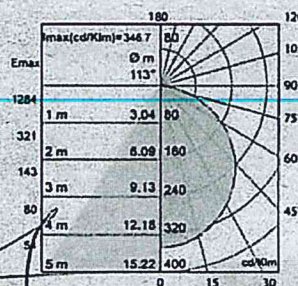
FOTOMETRIAS
