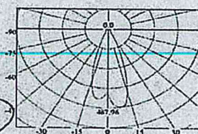
FOTOMETRIAS
