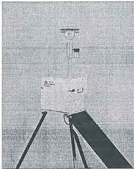
Muestreador Ambiental PM10 y PM2.5 PQ 200 con Panel Solar
