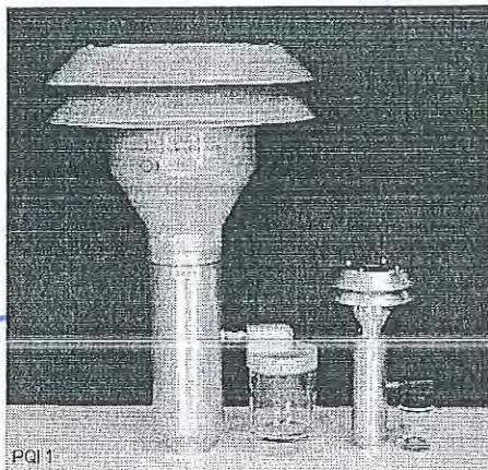
Entrada designada por la EPA y Entrada de Gran Altitud miniPM
